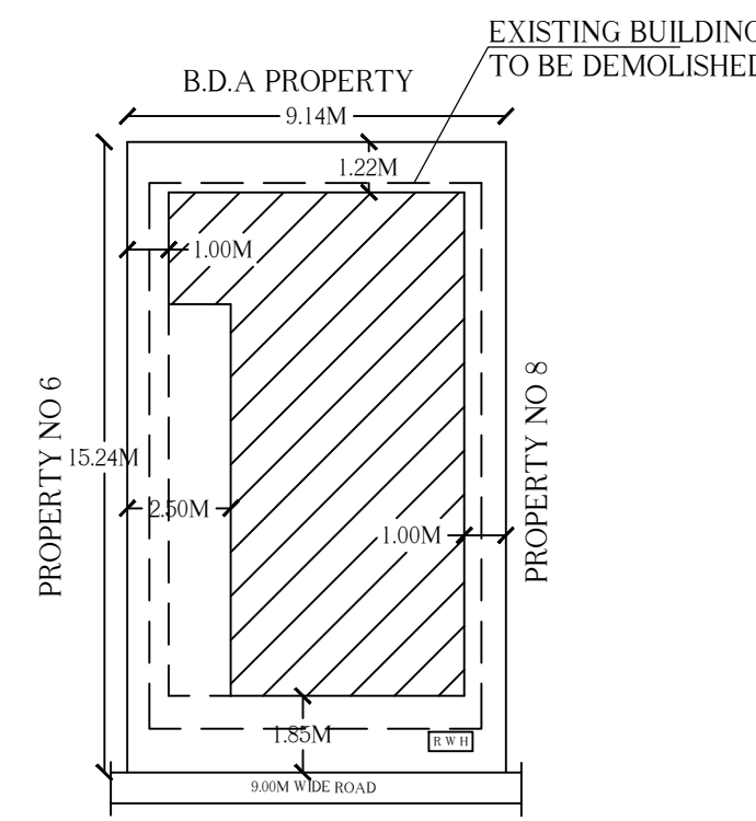
SITE PLAN 1:200
